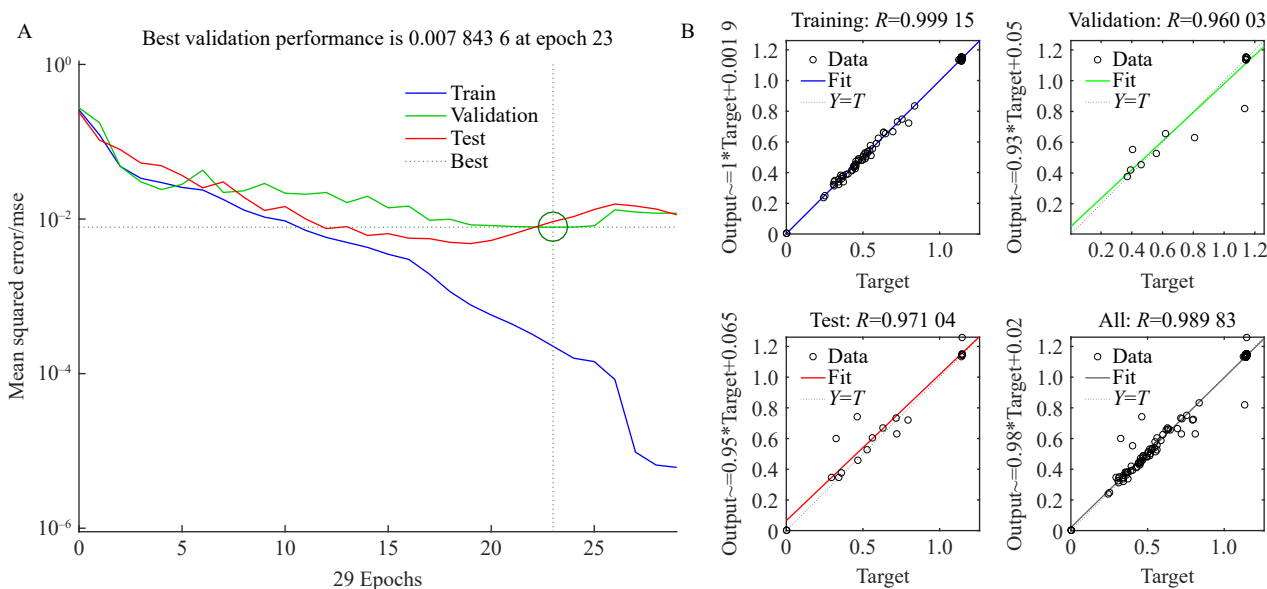
图 1 LM 算法构建的 BP 神经网络模型
